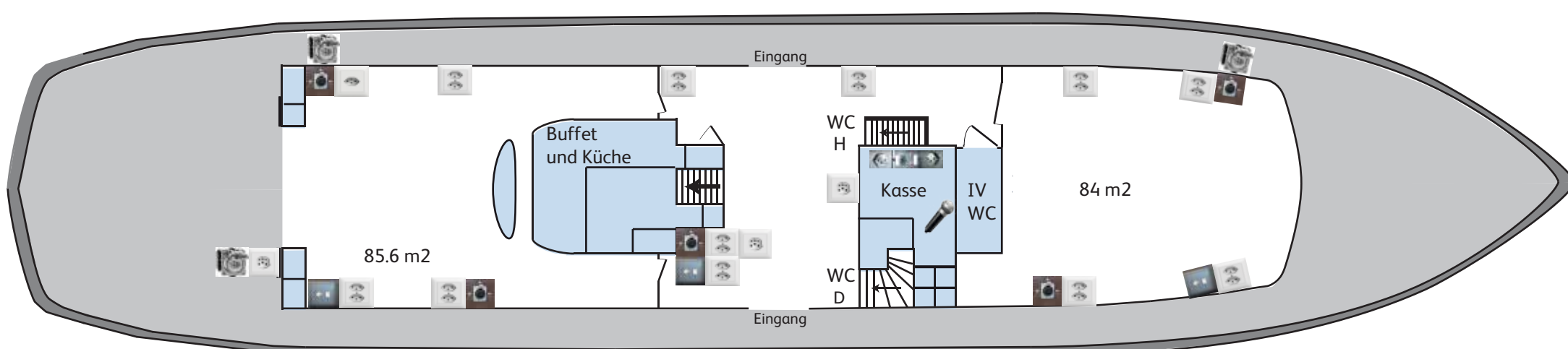
Hauptdeck
