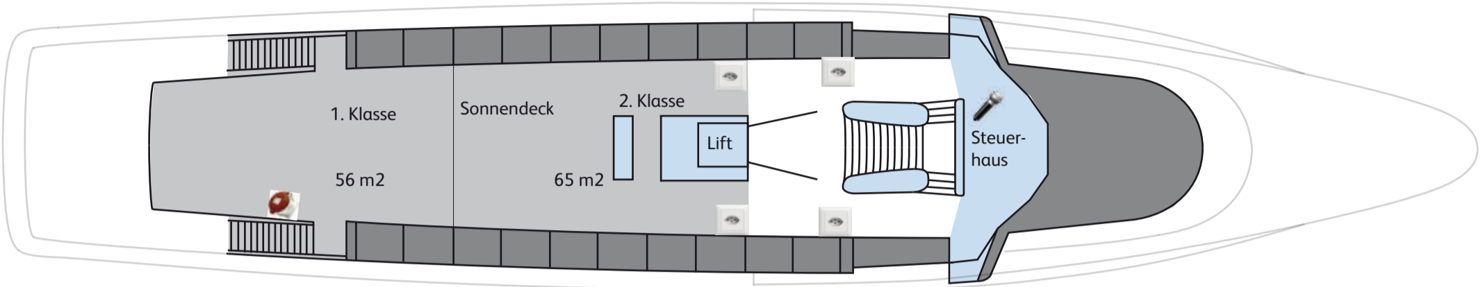
Sonnendeck
